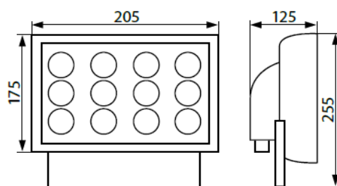
ALIX POWER LED12
